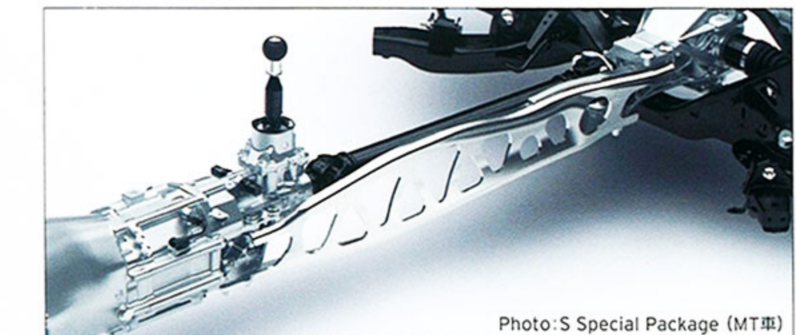
■パワー・プラント・フレーム[アルミ製](PPF)
